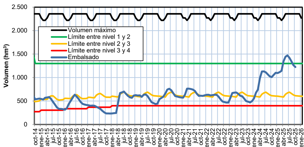
Figura 4. Niveles característicos y volúmenes embalsados a primeros de mes en el sistema Entrepeñas-Buendía desde octubre de 2014 1112 .
