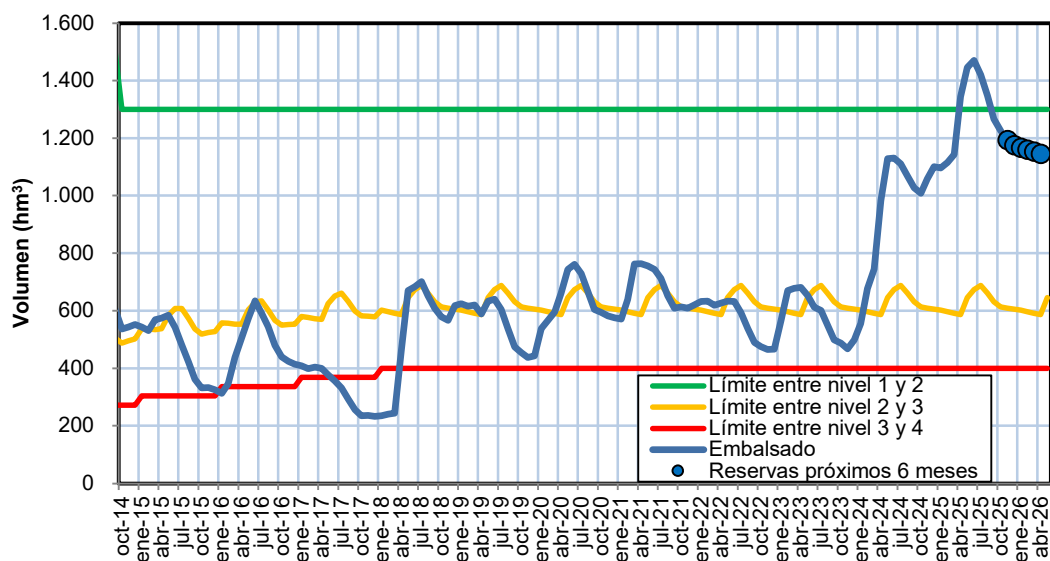
Figura 9. Evolución de las reservas en Entrepeñas-Buendía y reservas de cálculo para los próximos seis meses 13 14 .
